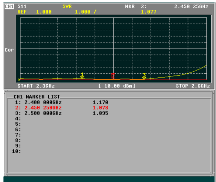
V.S.W.R
