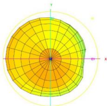
Total_3D_Front View_428MHz
