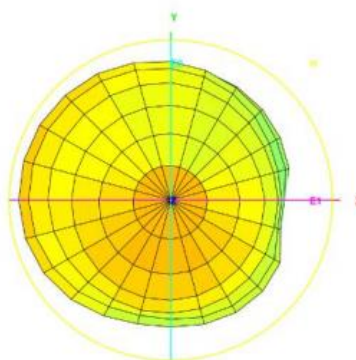
Total_3D_Front View_433MHz
