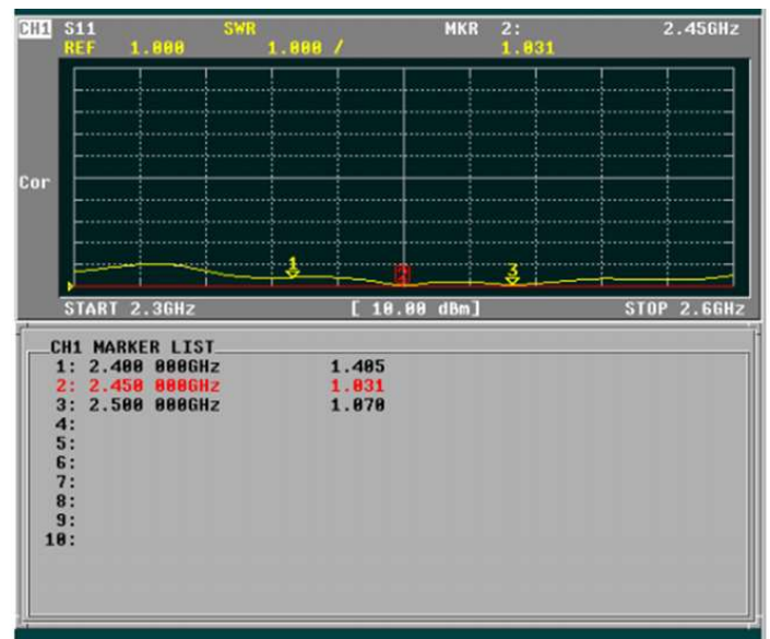
V.S.W.R
