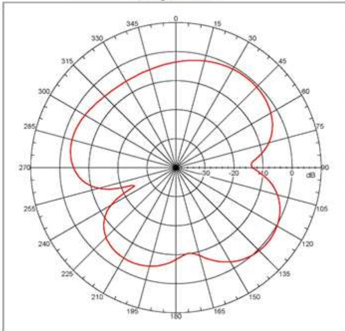
H-plane
