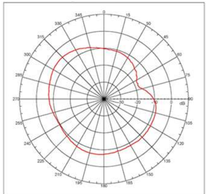
E-plane
