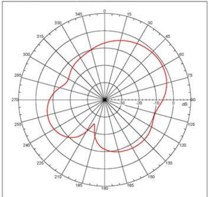
E-plane
