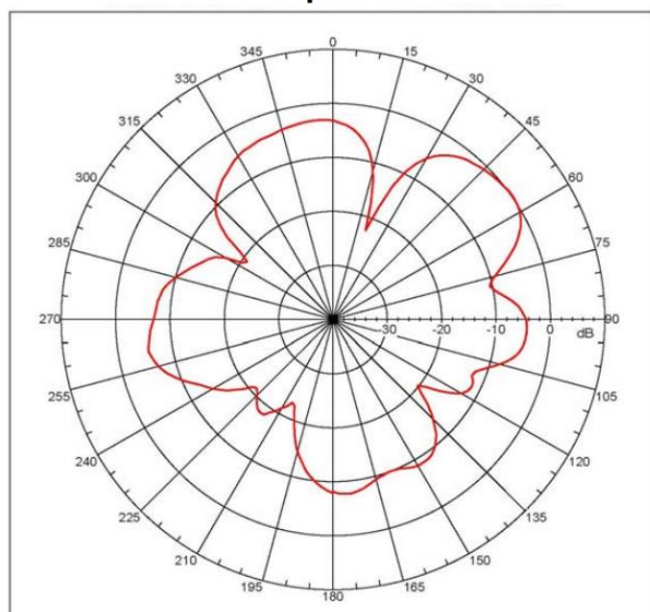
E-plane
