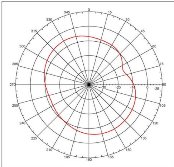
H-plane
