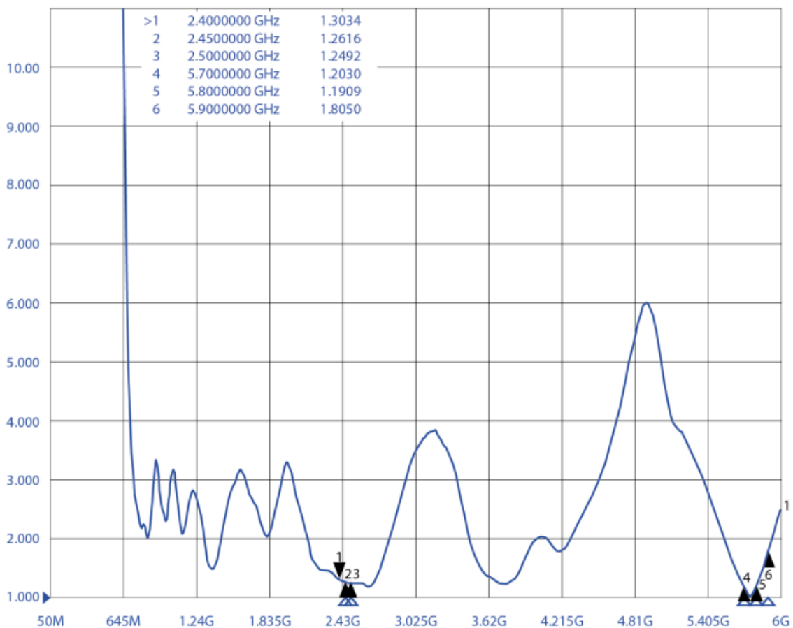
Tr1 S11 SWR 1.000/ Ref 1.000
