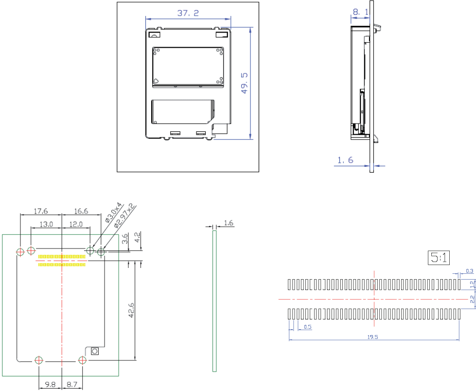
Module Clip PCB Footprint
